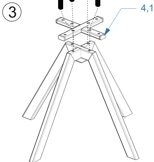
Прикрутить винтами(3) монтажную крестовину №2
