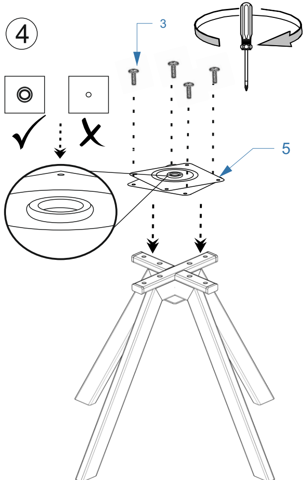
Установить поворотный механизм(большим кольцом вверх)
