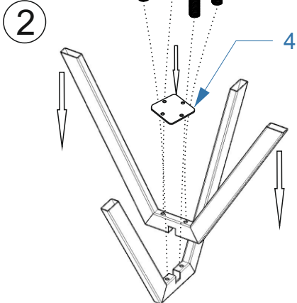
Соединить опоры между собой в паз, Прикрутить винтами(3) монтажную пластину №1
