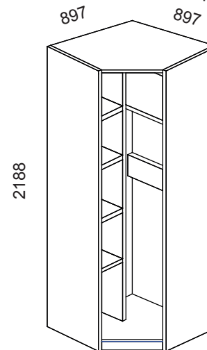
Каркас шкафа углового ТД 297.07.03 ПМ-297.09.00.000
