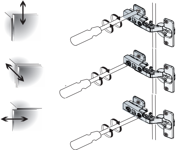
Регулировка петли
